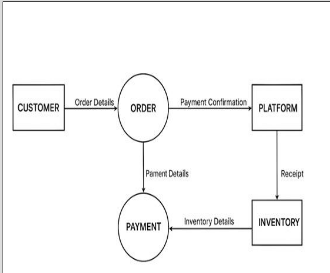
DFD Level-0
