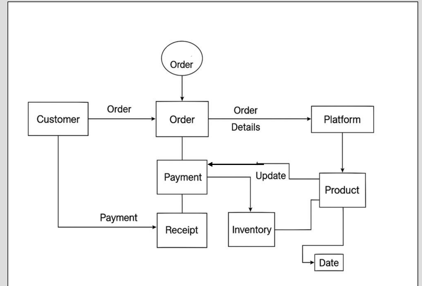
DFD Level-1
